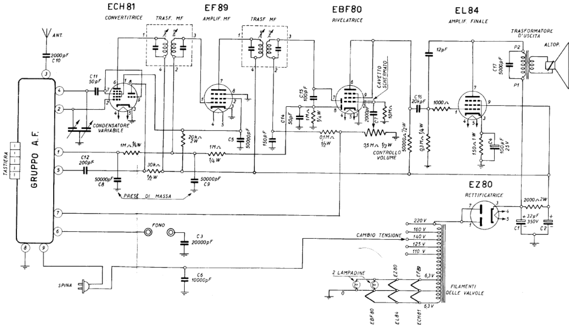
— Schema dell'apparecchio « Modulina AM ».
